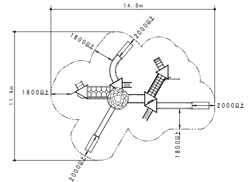
安全領域 平面図 1/200
