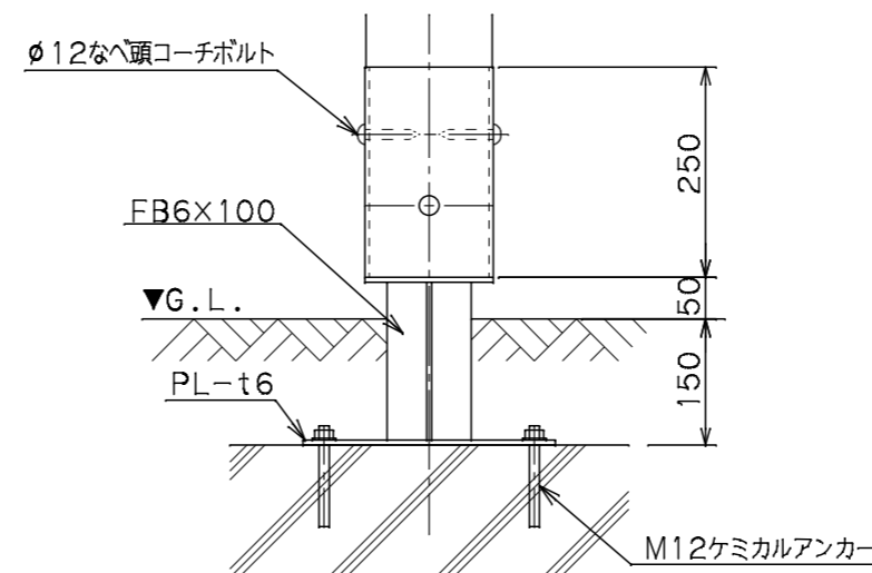
ベース金具詳細図 S=1/10 (金具部は溶融亜鉛メッキ・無塗装)
