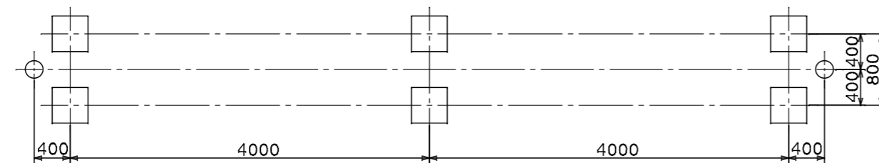
基礎伏図
