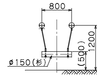
C-C矢視図
