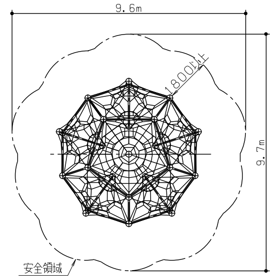
安全領域 平面図 1/150
