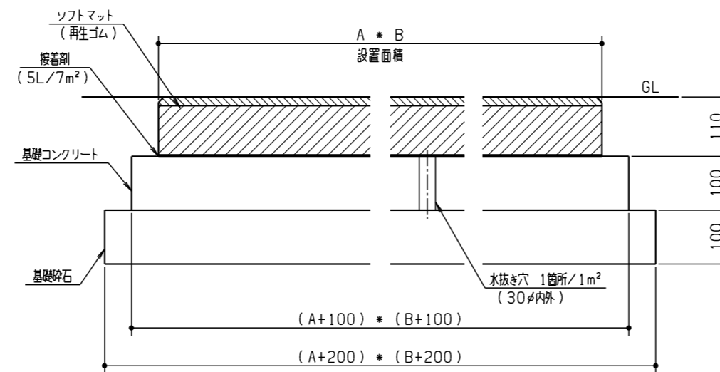
基礎凡例
