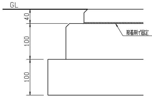
詳細図 1/5
