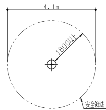
安全領域 平面図 1/100
