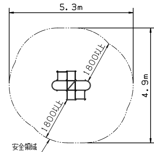
安全領域 平面図 1/100
