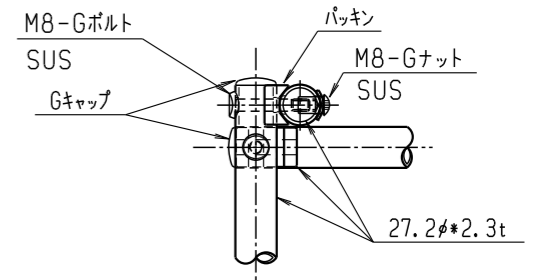
接合部 1/5
