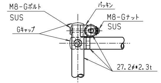
接合部 1/5
